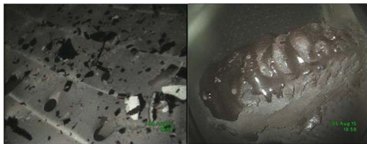
Fig.4.6-1 火山灰吸い込み試験後の燃焼器（左）とタービン翼（右）の写真 4.6.4)
